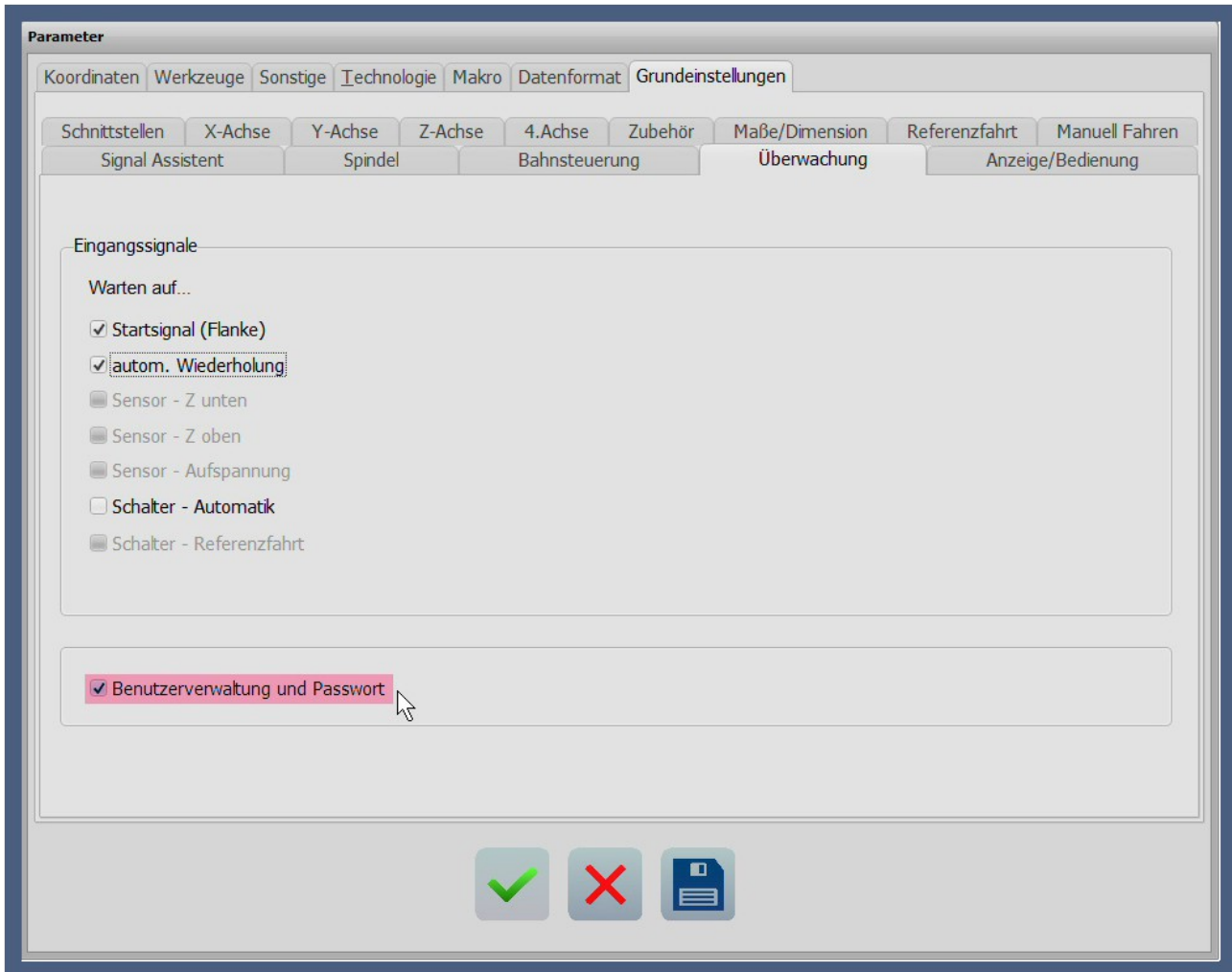
Aktivierung der Benutzerverwaltung
