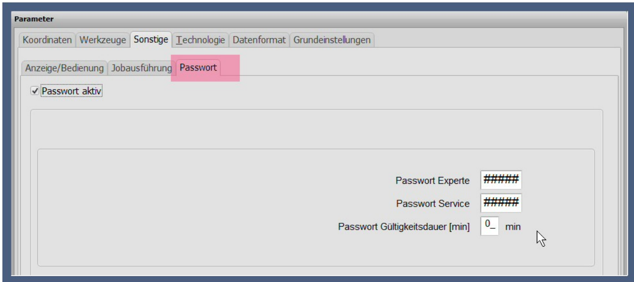
Passwortdialog
