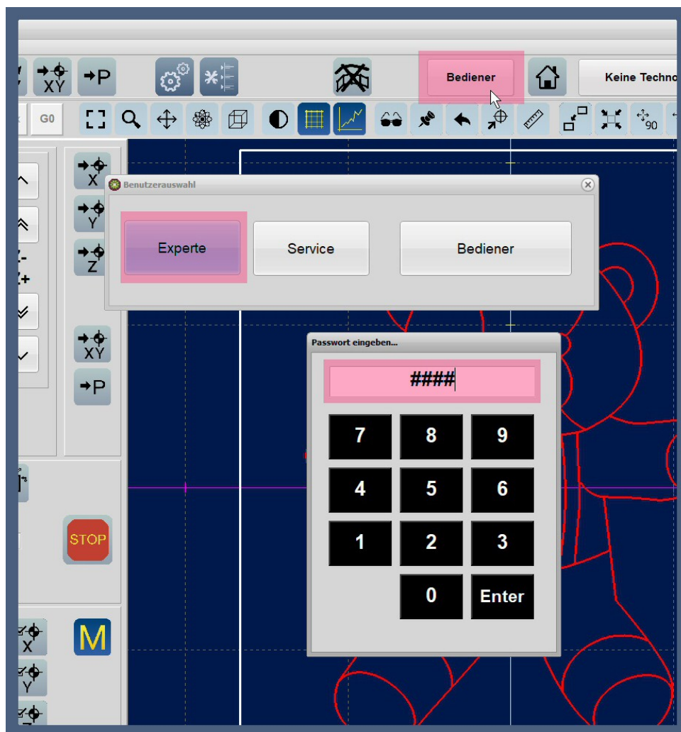
Verdeckte Passwordeingabe
